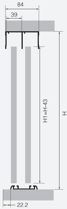
Aluminium frame door
